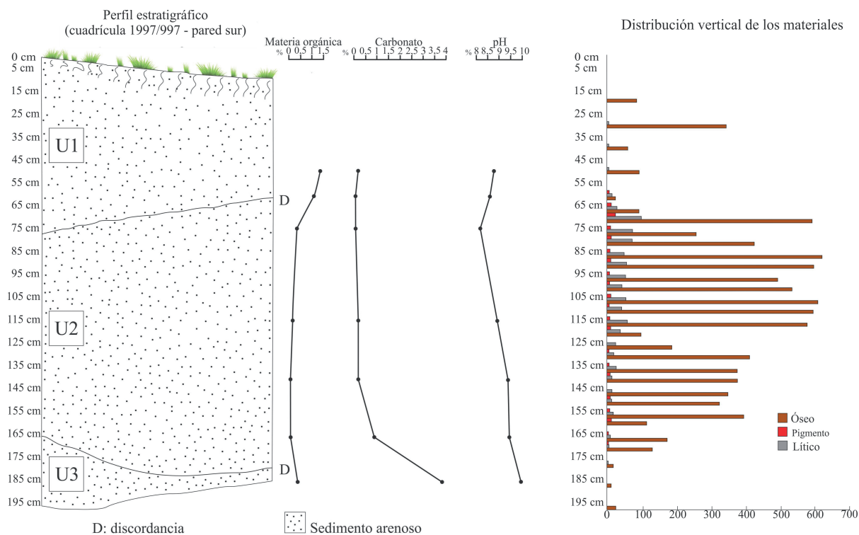
Figura 2. Estratigrafía de TO5.
